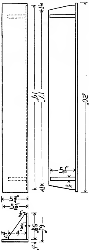
Fig. 162—Mantel Shelf
